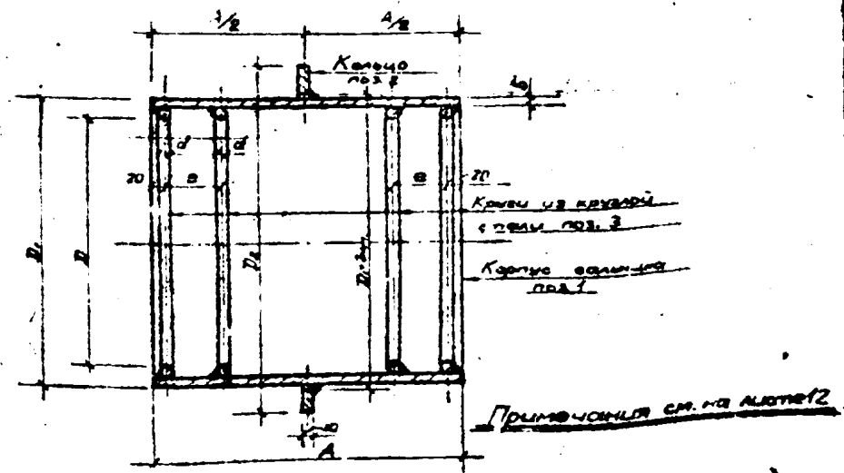
Корпус сальника, тип II (при A > 400\text{ мм} )
