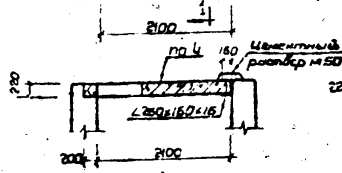
1-1 Колодцы 2100x2100 (Схема 1)
