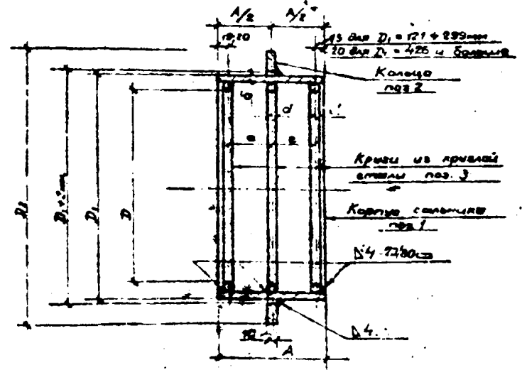
Корпус сальника, тип I (при A \le 400\text{ мм} )
