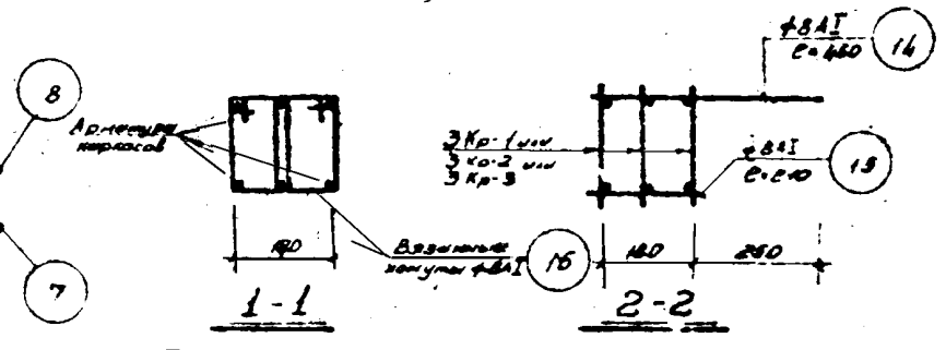
Деталь сварки плоских каркасов Kp-2 и Kp-3 в пространственный каркас.
