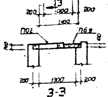
Колодцы 1300x1000 (схема 7)
