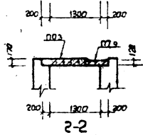
Колодцы 1300x300 (схема 6)
