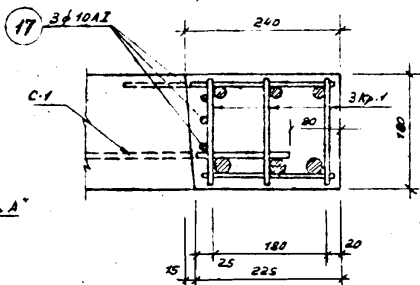
Узел А
