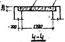
Колодцы 2100x1700 (схема 10)
