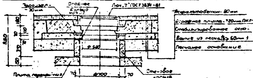
Тип III. Горловина люка для временной нагрузки H=80
