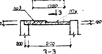
3-3 Колодцы 2100x1300 (Схема 3)
