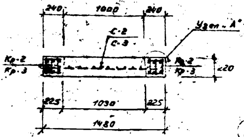
1-1 армирование
