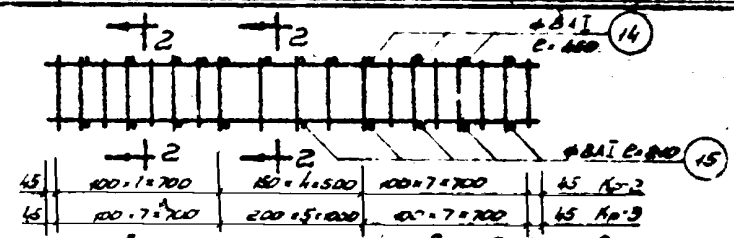
Деталь сварки плоских каркасов Kp-2 и Kp-3 в пространственный каркас.
