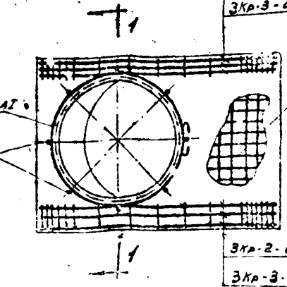
План ПК-2; ПК-3 / армирование /
