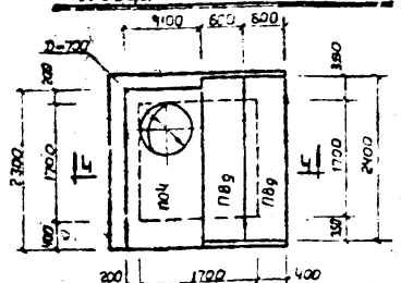
4-4 Колодцы 2100x1700 (Схема 4)
