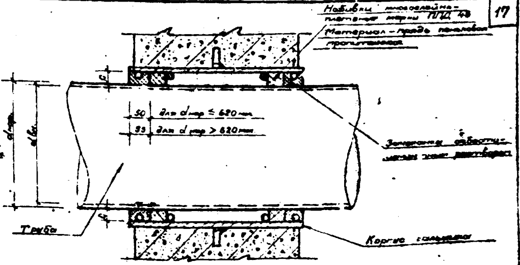
Узел установки сальника типа II
