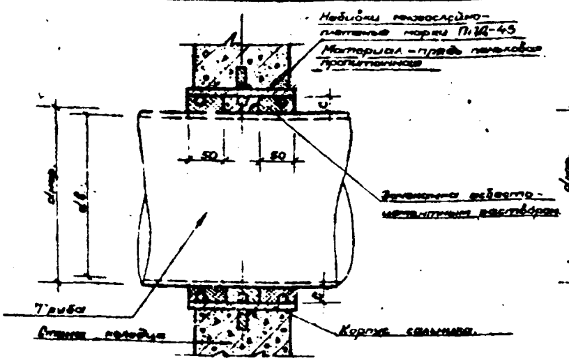
Узел установки сальника типа I
