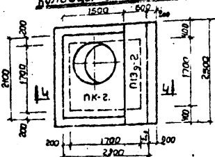
Колодцы 1700x1700 (схема 12)
